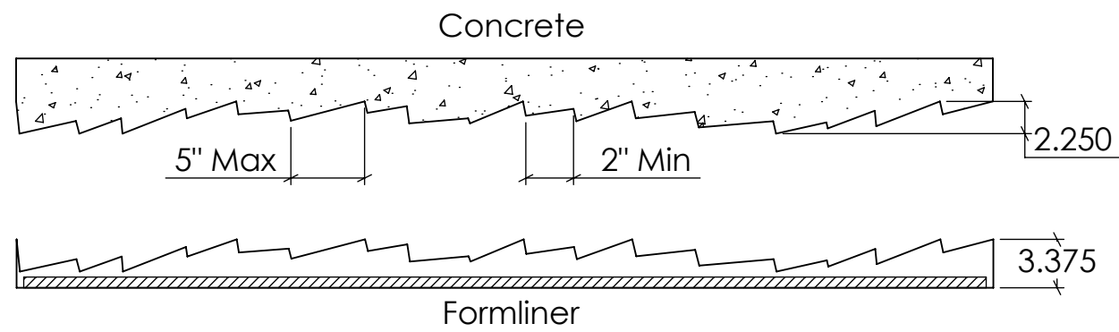
SECTION A-A SCALE 1 : 12
