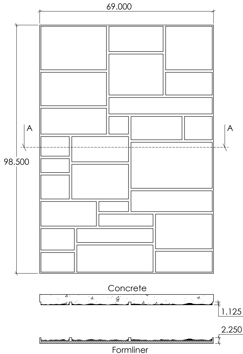
SECTION A-A SCALE 1 : 18
