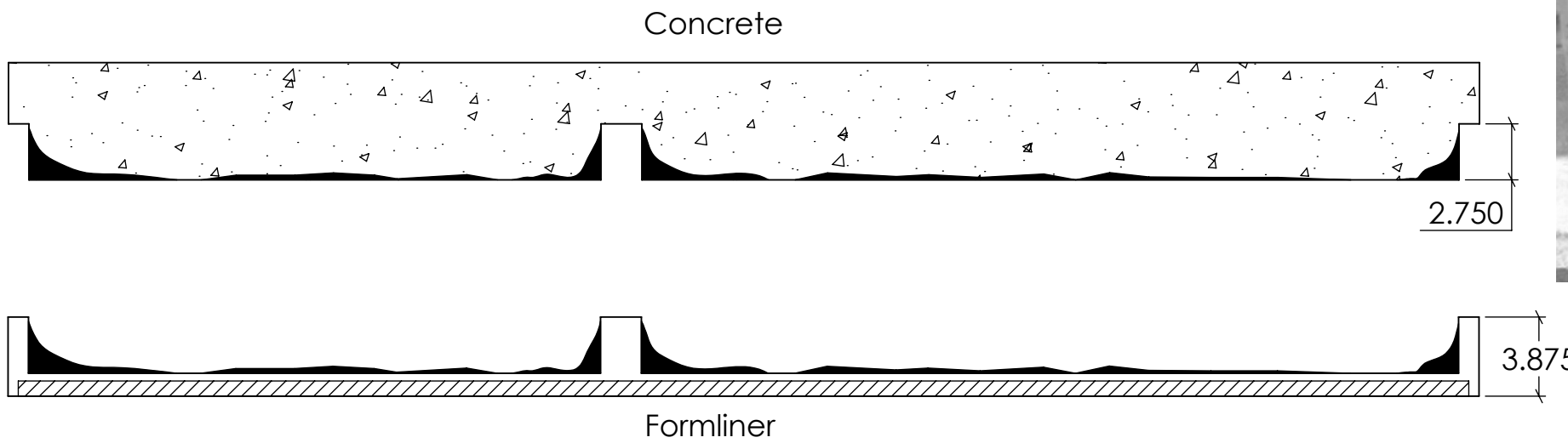
SECTION A-A SCALE 1 : 8
